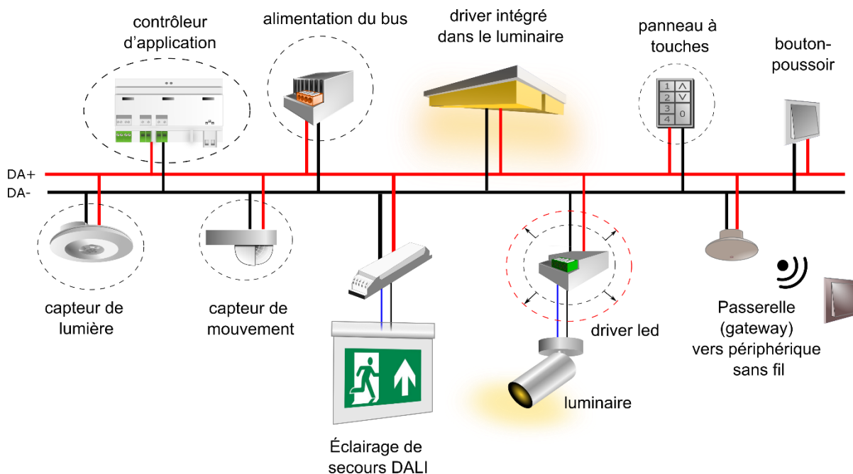
Figure 1 : exemple d'un réseau DALI typique avec des périphériques disponibles. Encerclées en pointillés, les pièces qui sont maintenant également incluses dans DALI-2 (le driver led a été réécrit)
