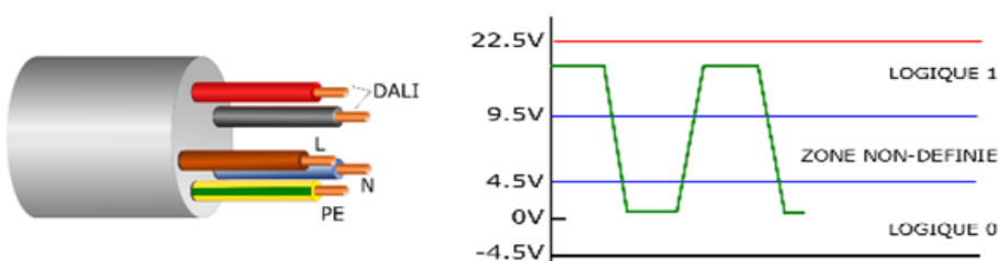
Figure 1 : Câblage typique et fluctuations en tension
